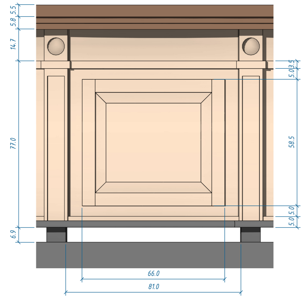
Elewacja baru ( 1 : 10 )
